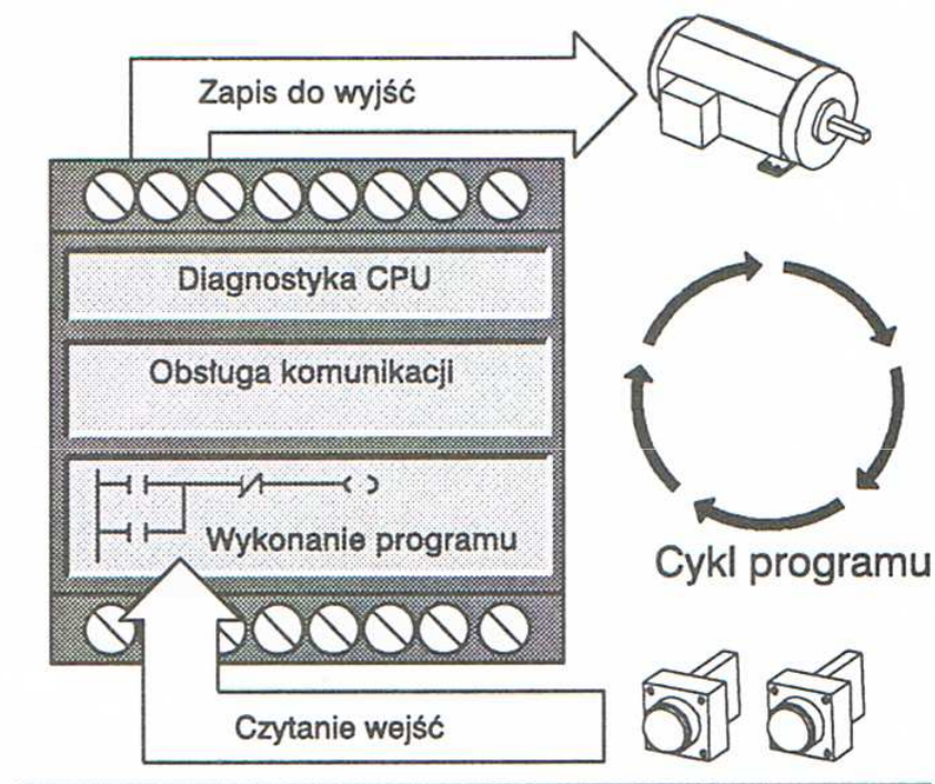
Rysunek 4-2 Cykl programu S7-200
